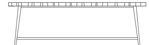
Dining Table VT90:160 h: 72 cm w: 90 cm l: 160 cm
