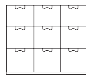
B3 9 drawers h: 84 cm d: 42 cm w: 90 cm
