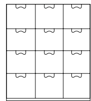
B 12 drawers h: 109 cm d: 42 cm w: 90 cm
